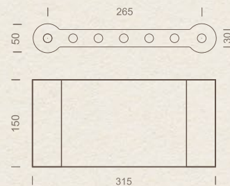
CURTAIN CYLINDER PIECE. PIEZA CURTAIN CILINDRO. PIÈCE CYLINDRE CURTAIN
